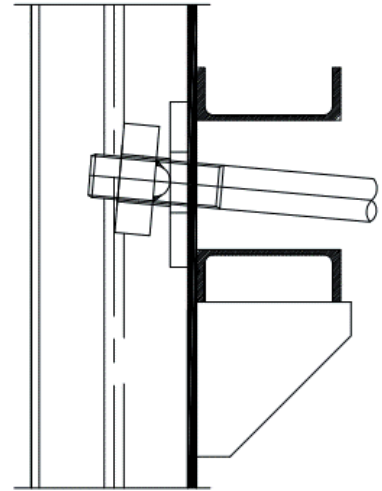
Rückverankerung U-Profile
